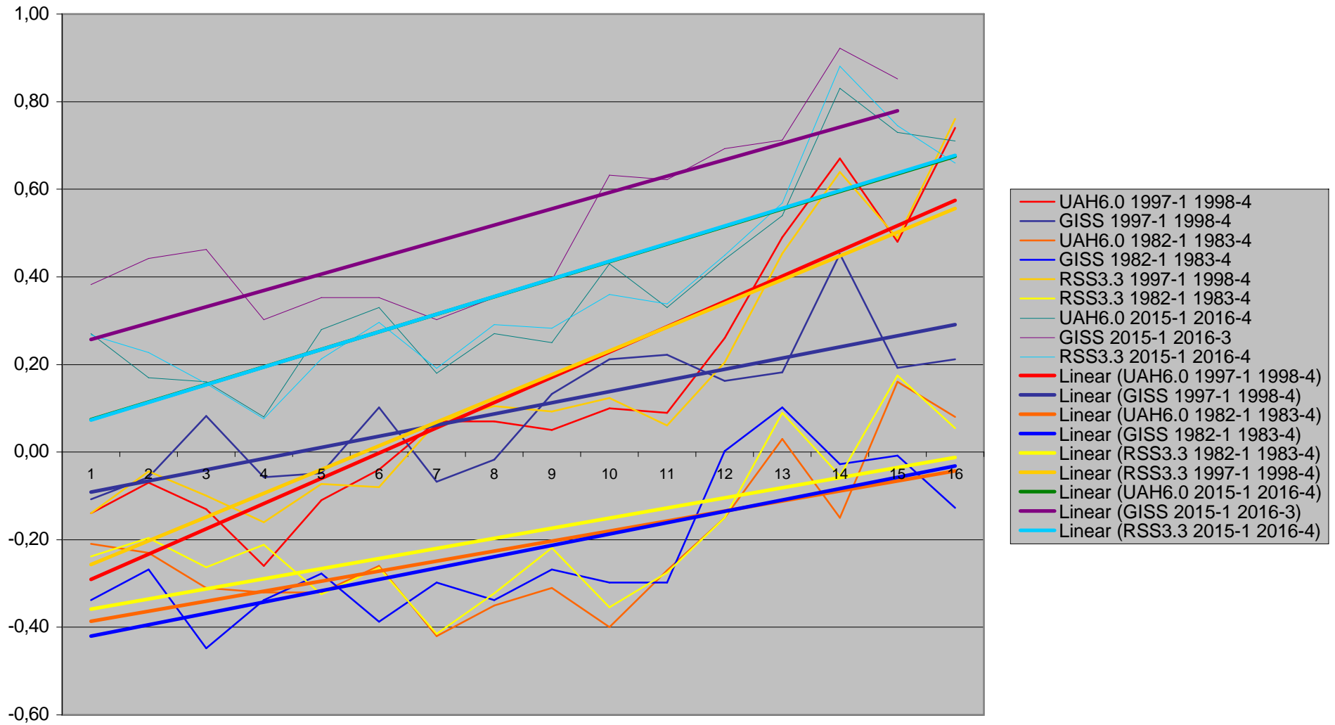
UAH6.0beta5 TLT / RSS3.3 TLT / GISS surf : El Niños 1982/83 - 1997/98 - 2015-16
