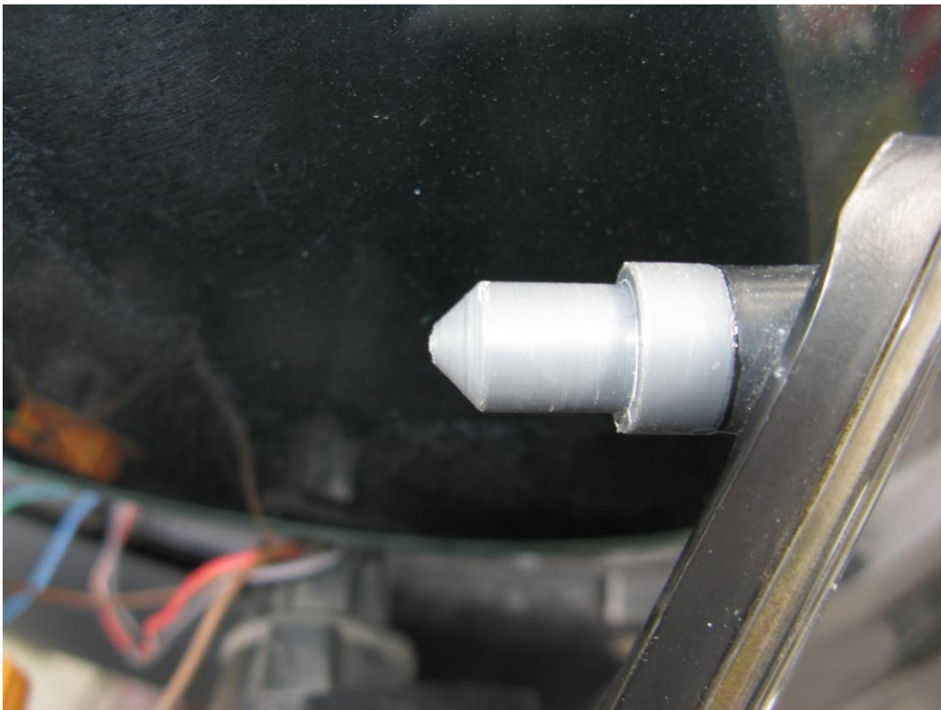
Smart Haltestift fürs Rücklicht mit Kunststoffkleber einkleben
